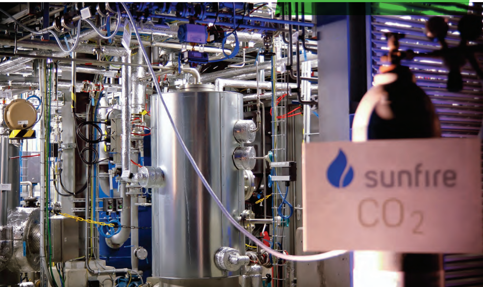
Produktionsanlage für Rohdiesel aus CO 2 , Wasser und Strom mit dem Verfahren der Fischer-Tropsch-Synthese
