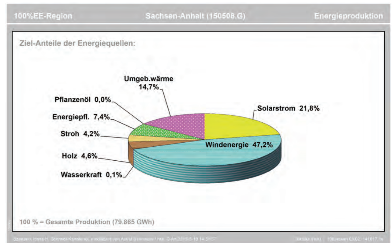
Anteile Erneuerbarer Energieproduktion im Zielszenario an Gesamtproduktion
