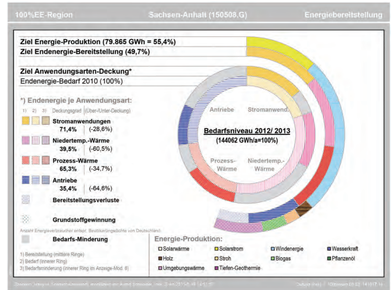
Kreise von innen nach außen: Energiebedarf heute, Ziel Energiebedarf und Ziel Bedarfsminderung (grau), Ziel Energiebedarf (zusammengeschobene Reststücke Bedarf), Ziel regenerative Energiebereitstellung zur Deckung des verbleibenden Energiebedarfes
